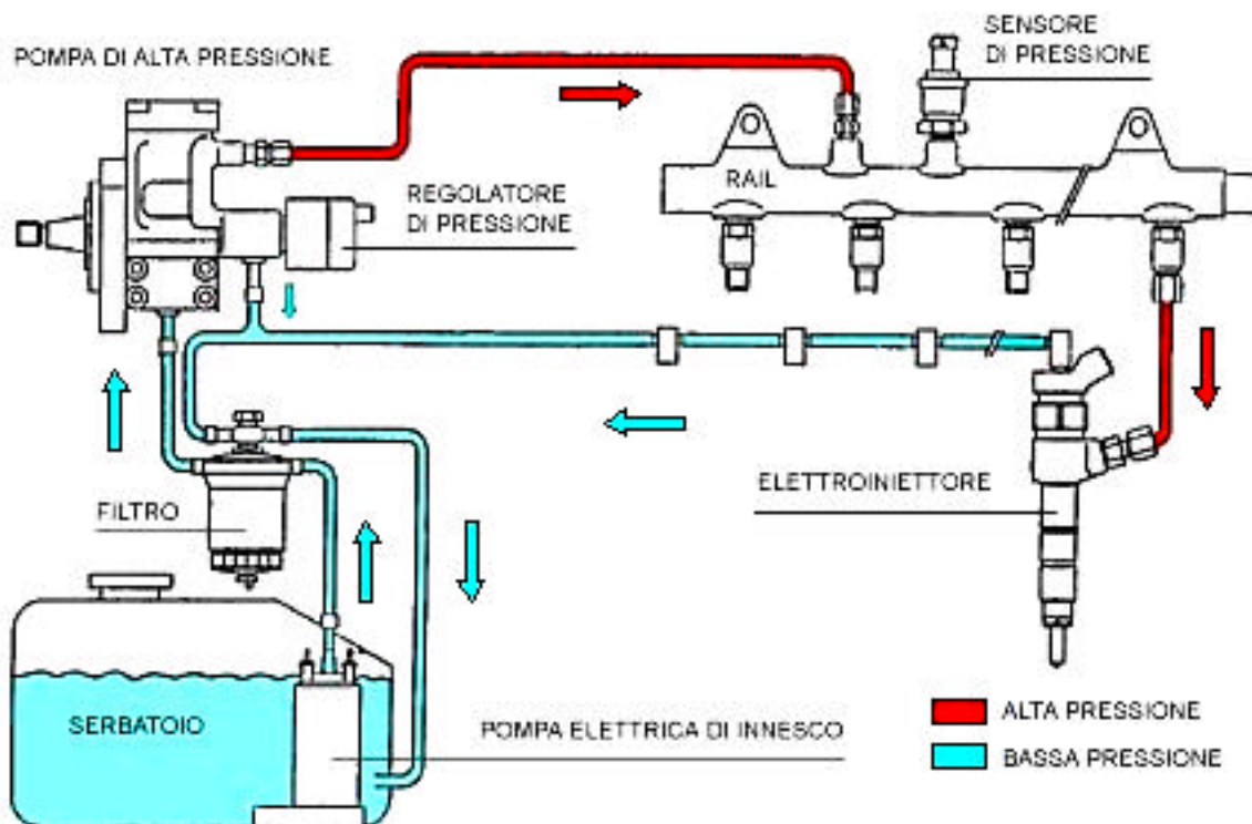
Figura 3 – Sistema di iniezione Common Rail: schema idraulico
