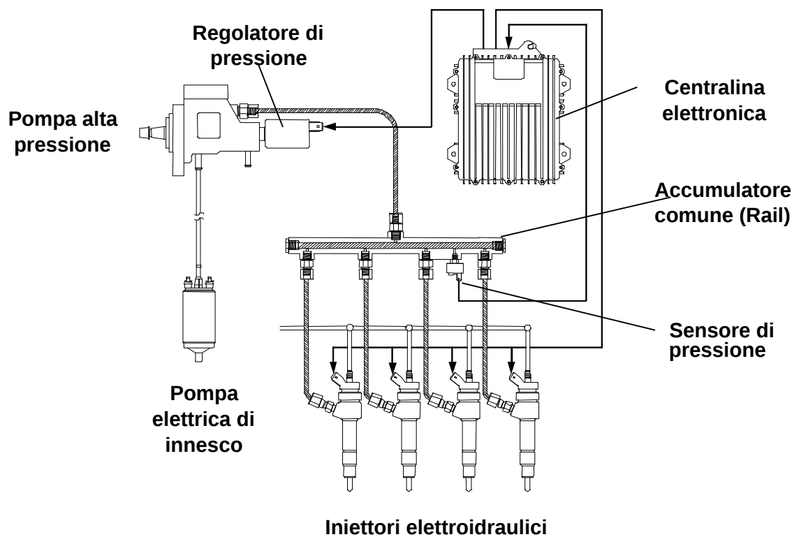
Figura 2 – Sistema di iniezione Common Rail: schema generale
