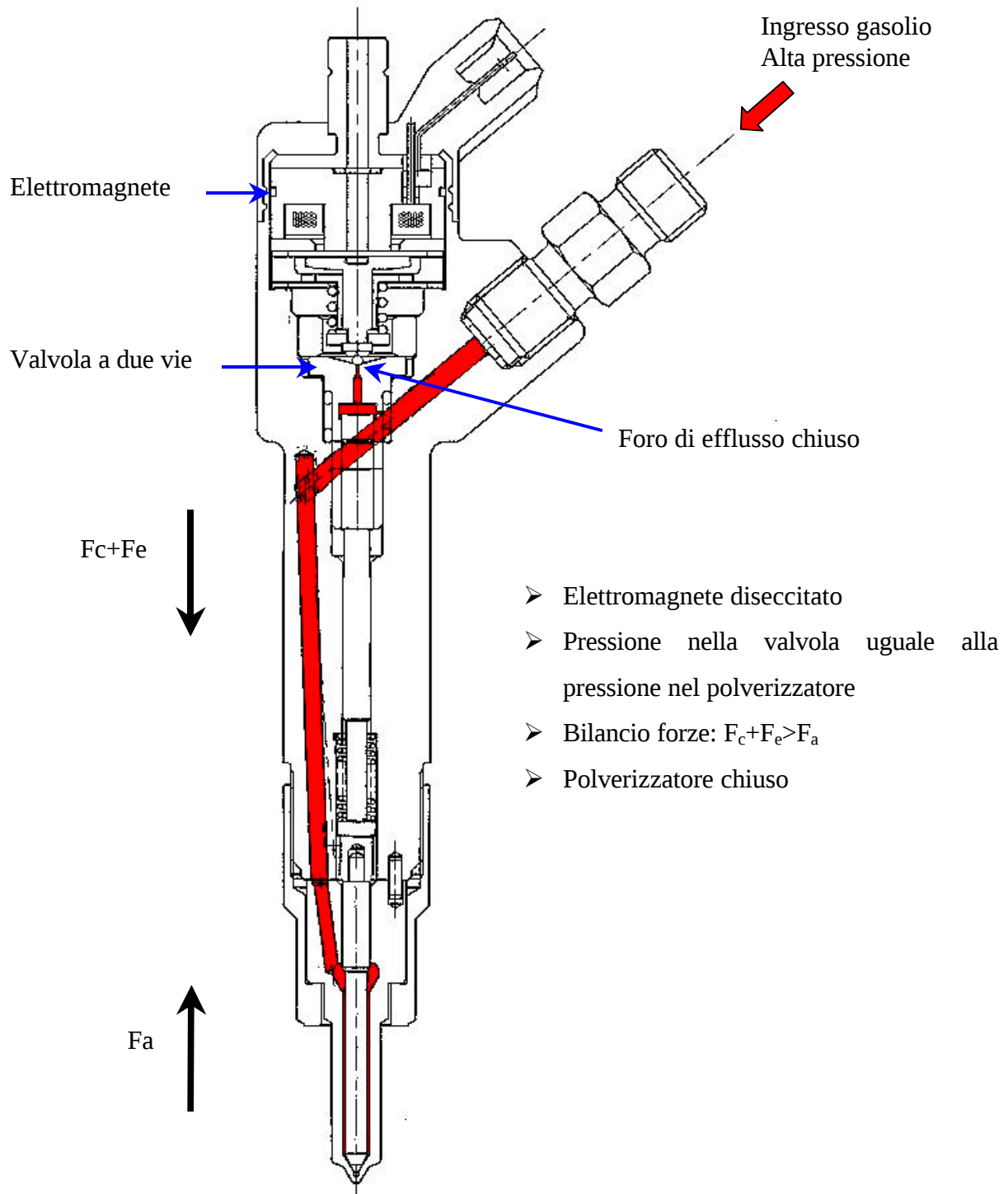
Figura 5 – Principio di funzionamento elettroiniettore: posizione di riposo
