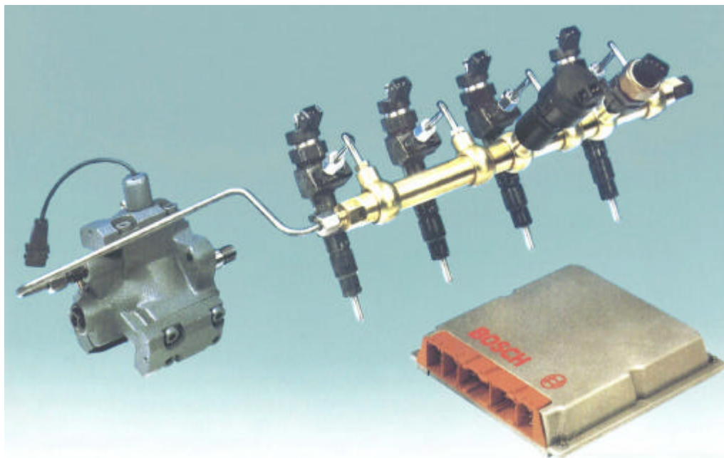
Figura 1 – Sistema di iniezione Common Rail
