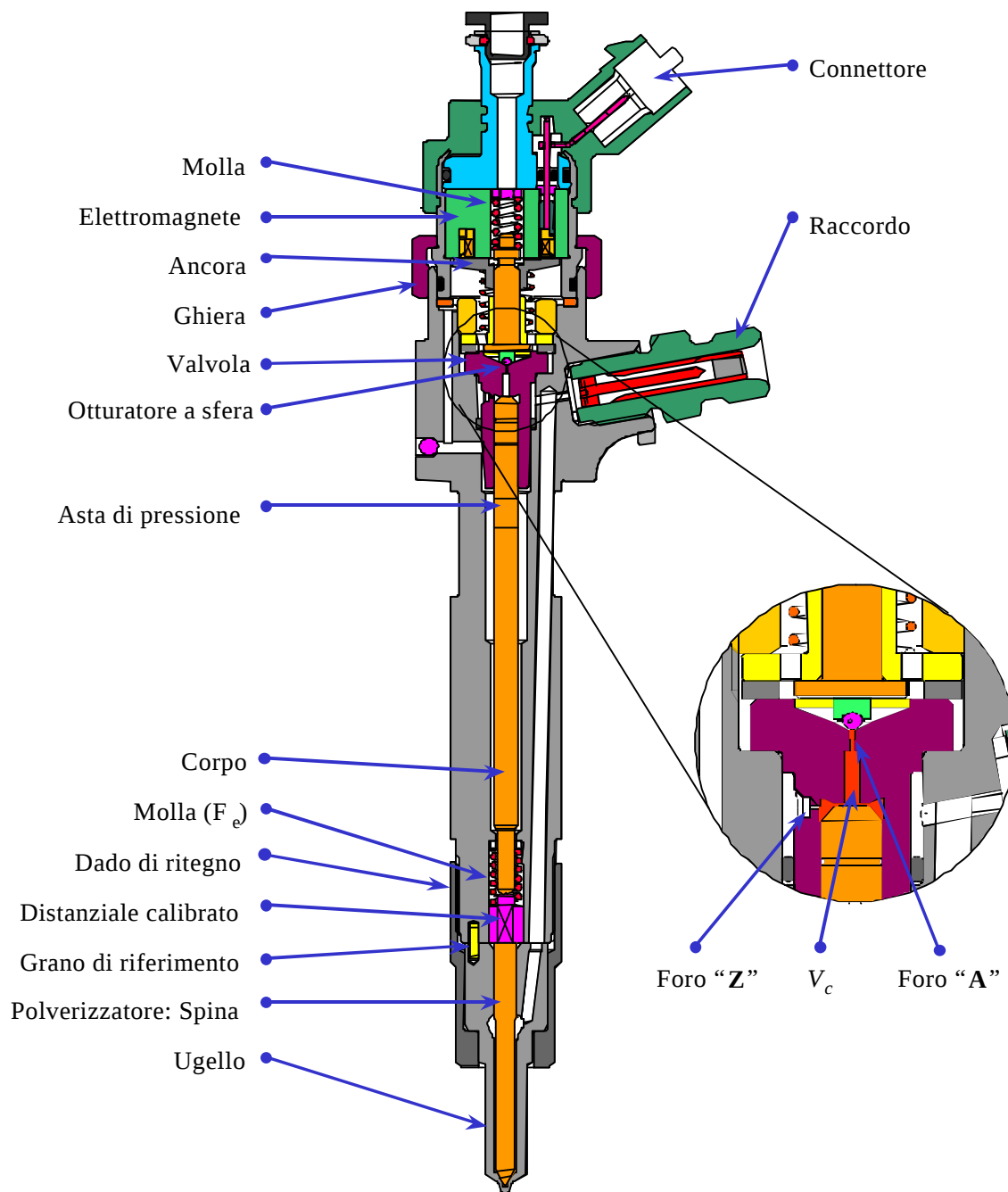
Figura 4 – Elettroiniettore
