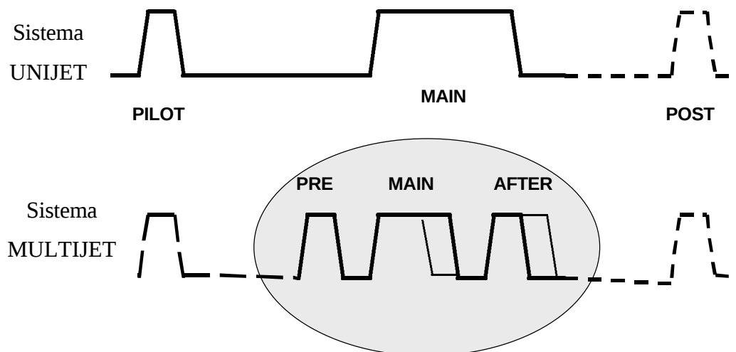
Figura 3.9 – Modalità di comando dell'iniezione realizzabili con sistema UNIJET e MULTIJET.
