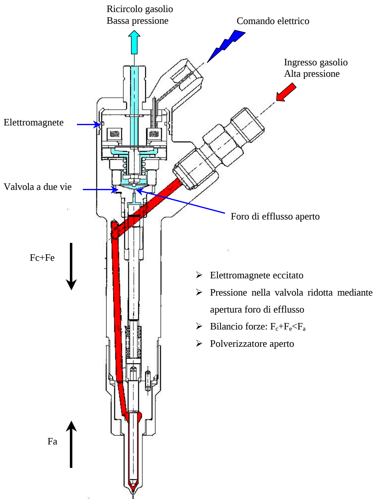
Figura 6 – Principio di funzionamento elettroiniettore: attuazione iniezione
