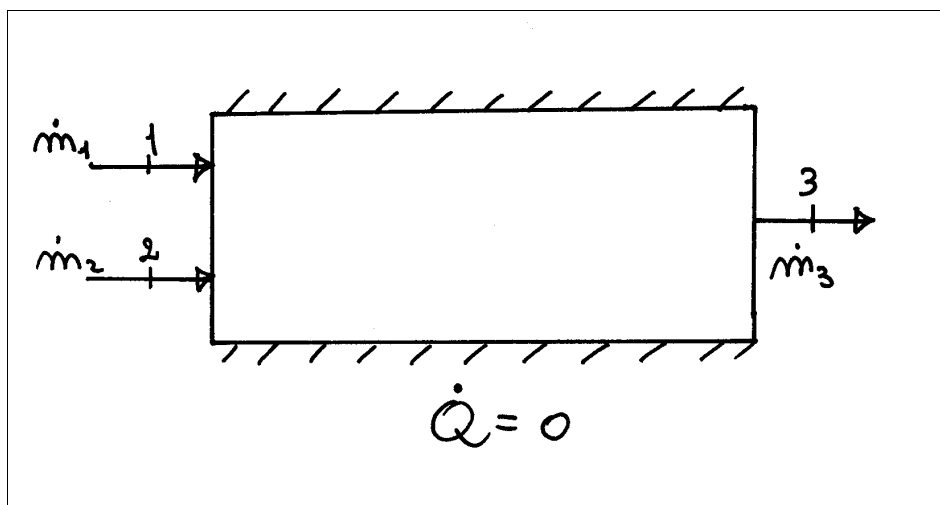
Fig. 3.6 - Schema di sistema aperto: condotto orizzontale con due ingressi ed un'uscita con pareti adiabatiche
