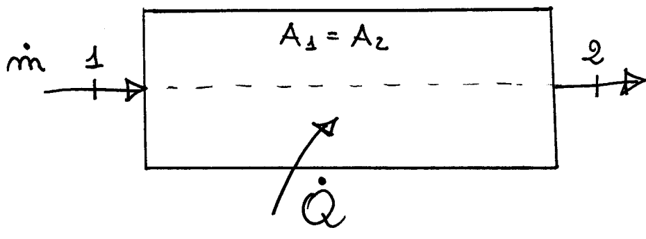
Fig.3.5 – Schema di sistema aperto
