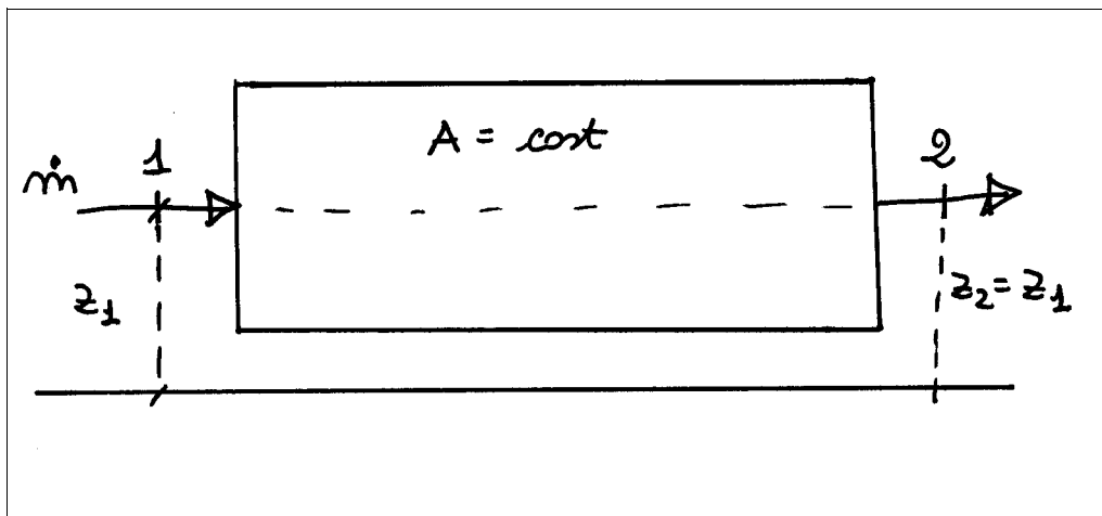
Fig. 3.1 - Schema di sistema aperto: condotta orizzontale a sezione costante
