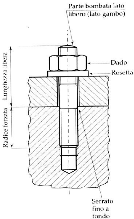
COLLEGAMENTO CON VITE PRIGIONIERA
