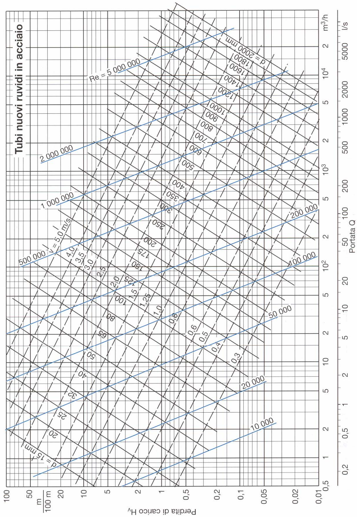
Fig. 11: Perdite di carico H_v per tubazioni nuove in acciaio ( k = 0,05 \text{ mm} )
