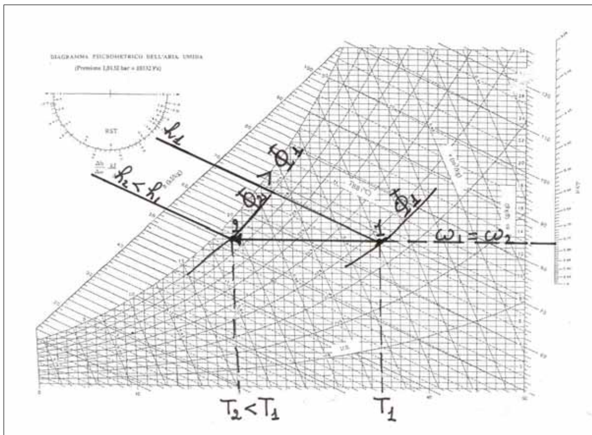
Fig.2.3.2.1 – Semplice raffreddamento
