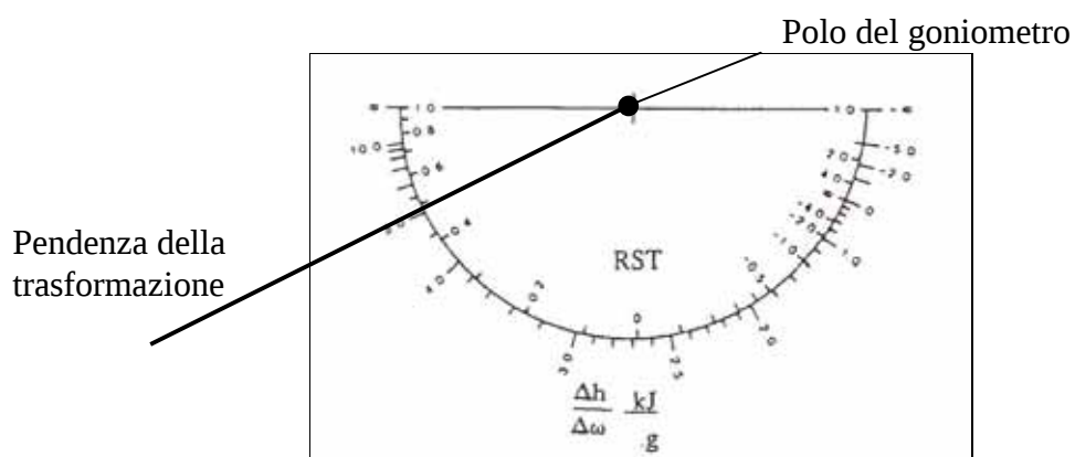
Fig.2.3.1 – Goniometro
