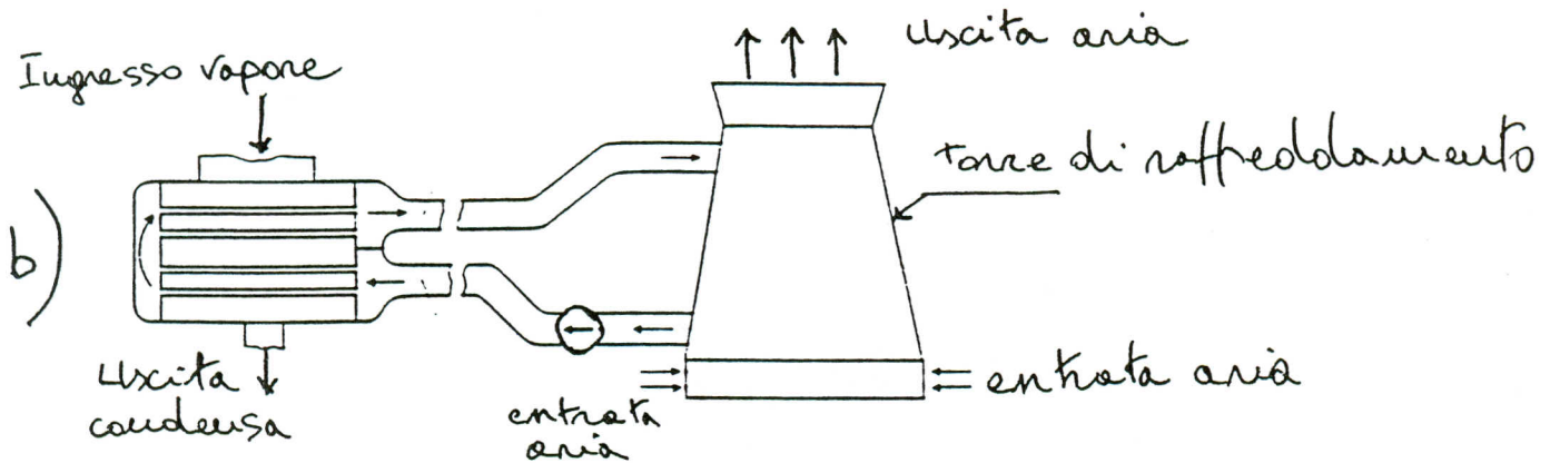
— Circuiti di raffreddamento per i condensatori: a) di tipo aperto; b) di tipo chiuso con torre di raffreddamento.
