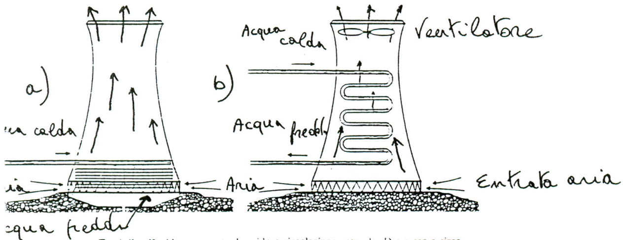
— Torri di raffreddamento: a) ad umido a circolazione naturale; b) a secco a circolazione forzata.
