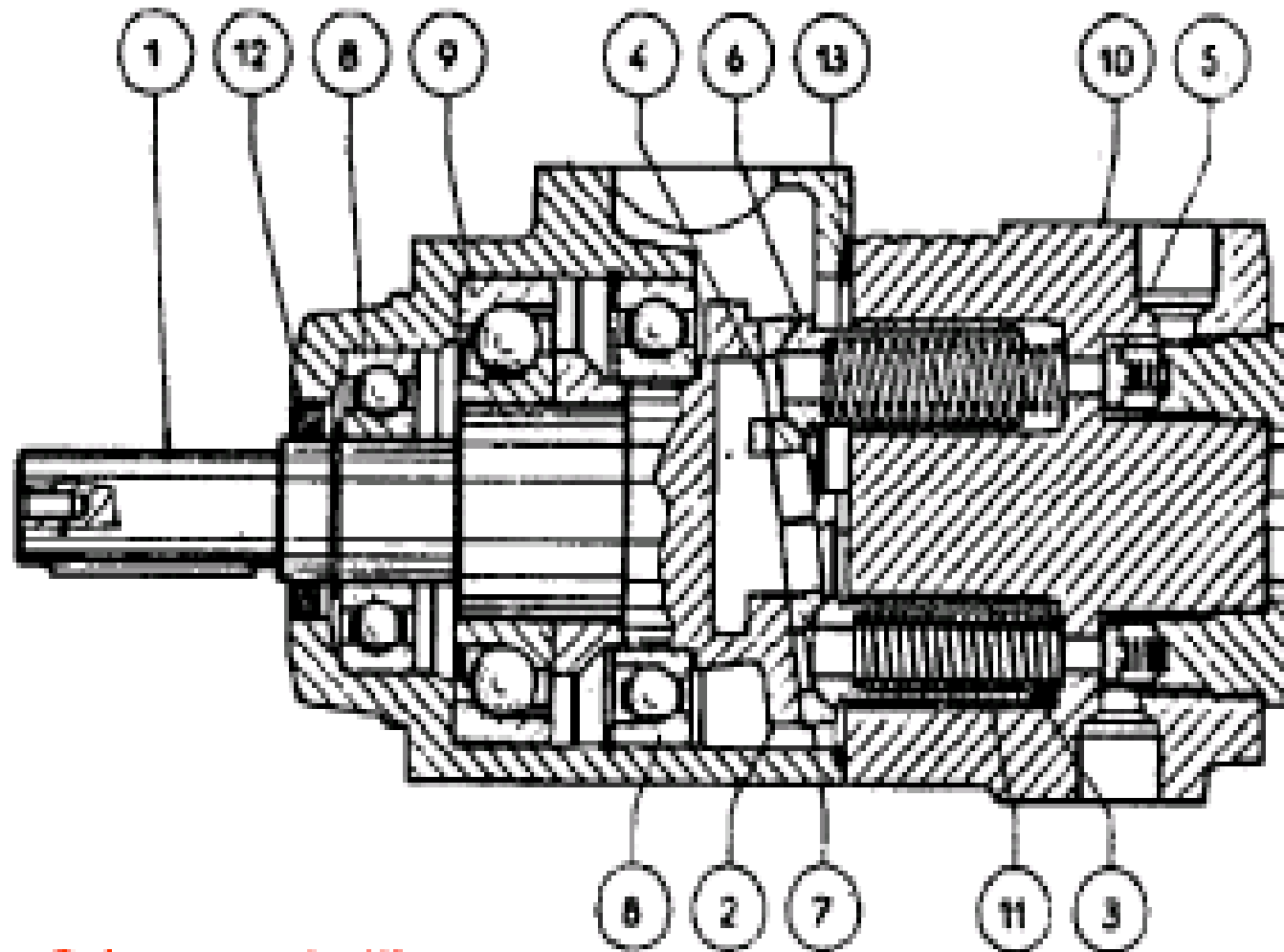
Schema costruttivo
